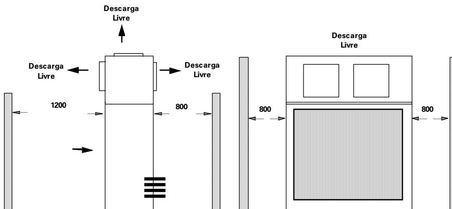
Fig. 42 - Espaços sugeridos para manutenção e circulação de ar. Unidade condensadora TRCE 050 a 150.
