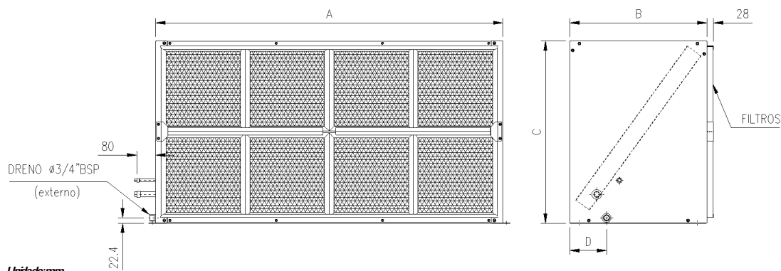
Fig. 20 - Dimensional Módulo Serpentina 350 a 500
