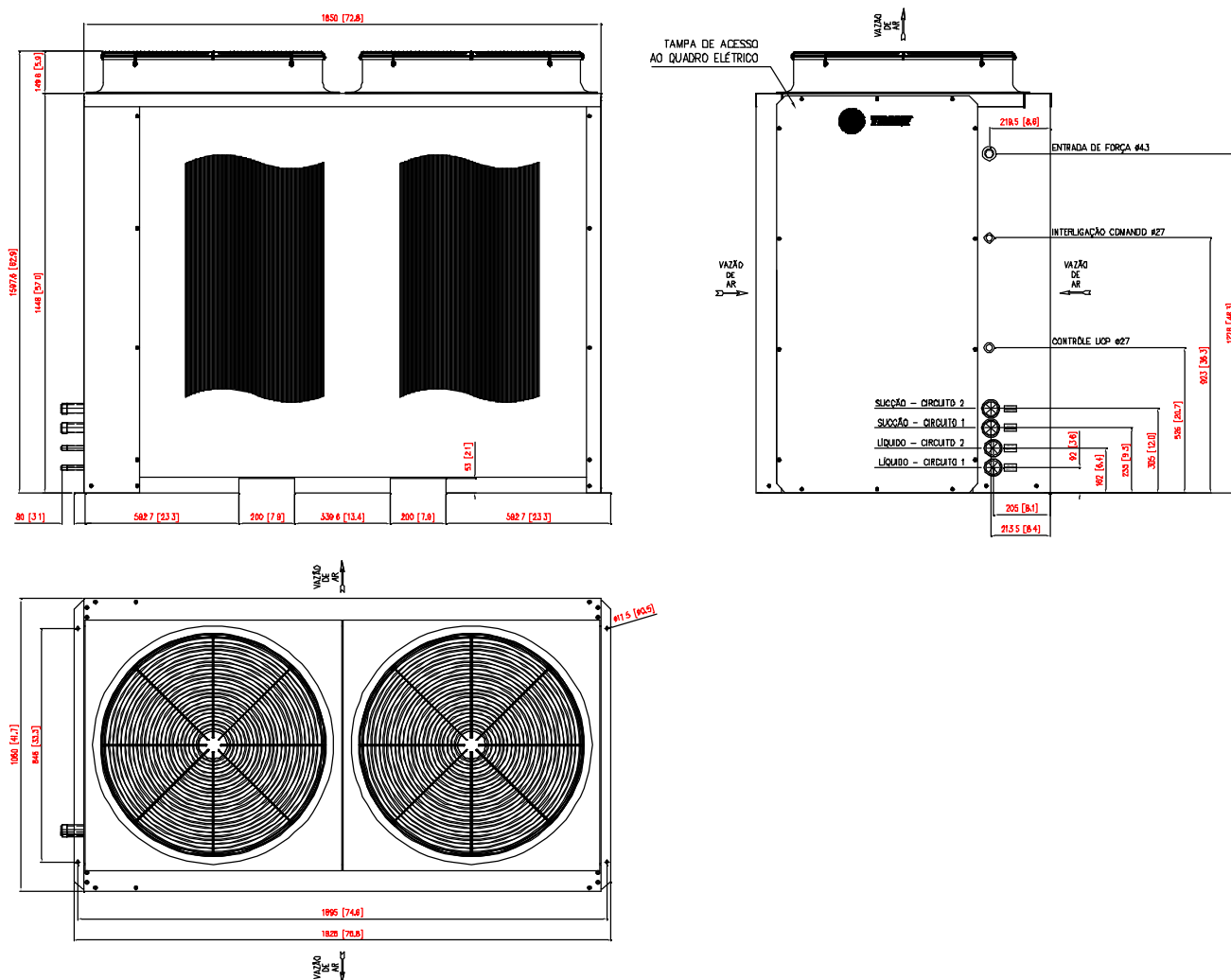
Fig. 40 - Dimensional Unidades Condensadoras TRAE 300 - 2 Circuitos
