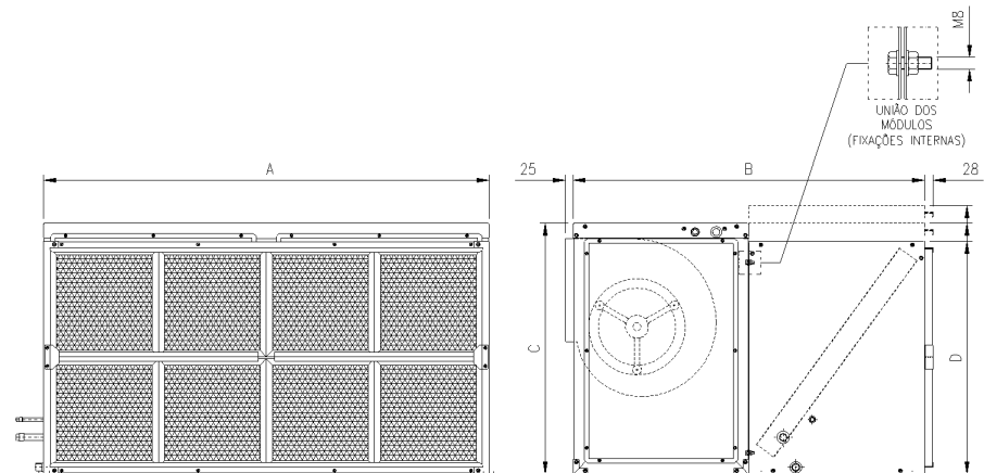
Fig. 23 - Montagem dos Módulos Ventilador e Serpentina CXPA 050 a 500 - Horizontal
