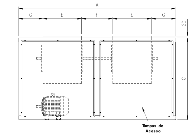
Fig. 15 - Dimensional Módulo Ventilador 200 a 300
