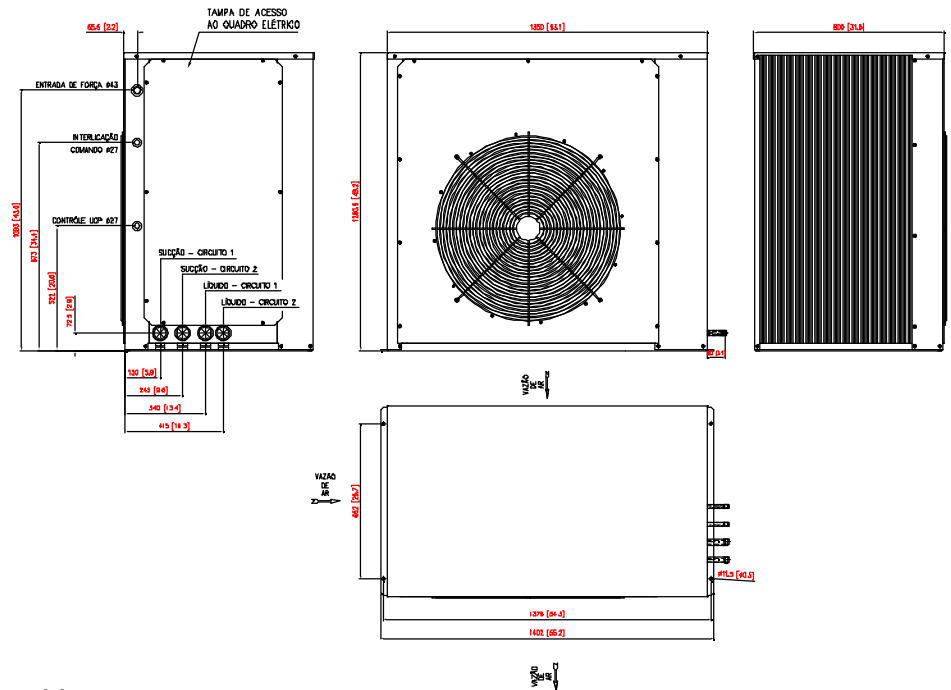
Fig. 33 - Dimensional Unidades Condensadoras TRAE 125
