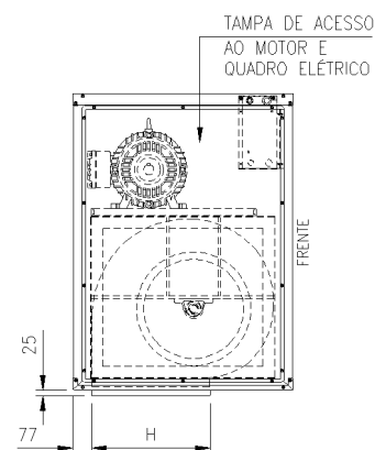
Fig. 19c - Descarga Piso
