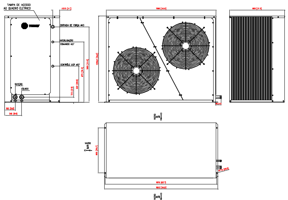
Fig. 34 - Dimensional Unidades Condensadoras TRAE 150 - 1 Circuito
