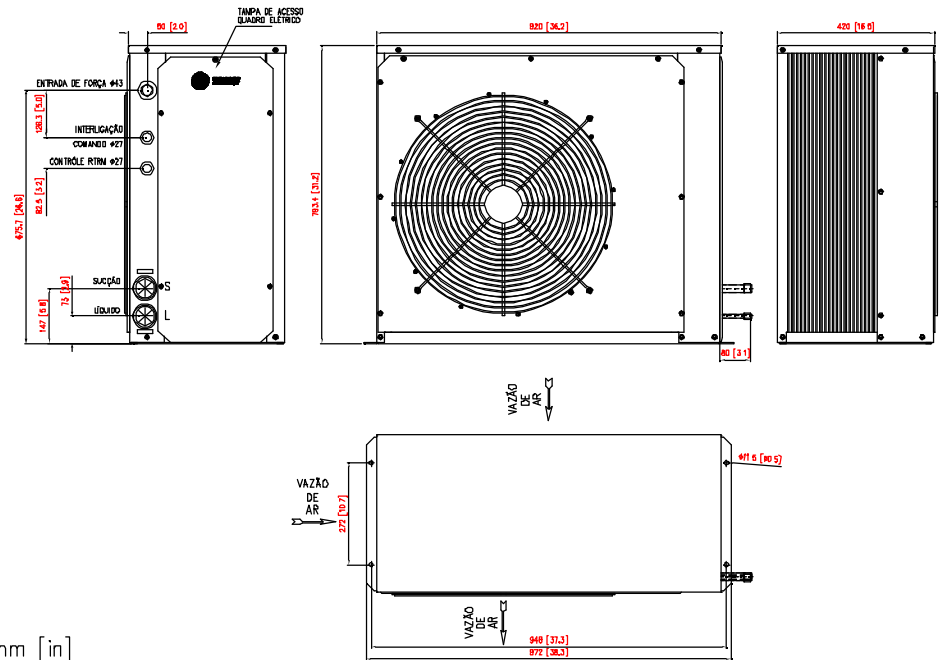
Fig. 29- Dimensional Unidades Condensadoras TRAE 050 1 circuito
