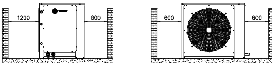
Fig. 41 - Espaços sugeridos TRAE 200 a 300 - Descarga Vertical
