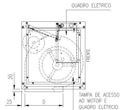
Fig. 10c - Descarga Piso
