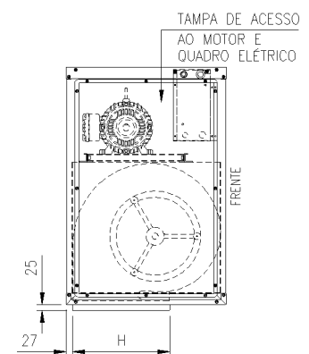
Fig. 16c - Descarga Piso
