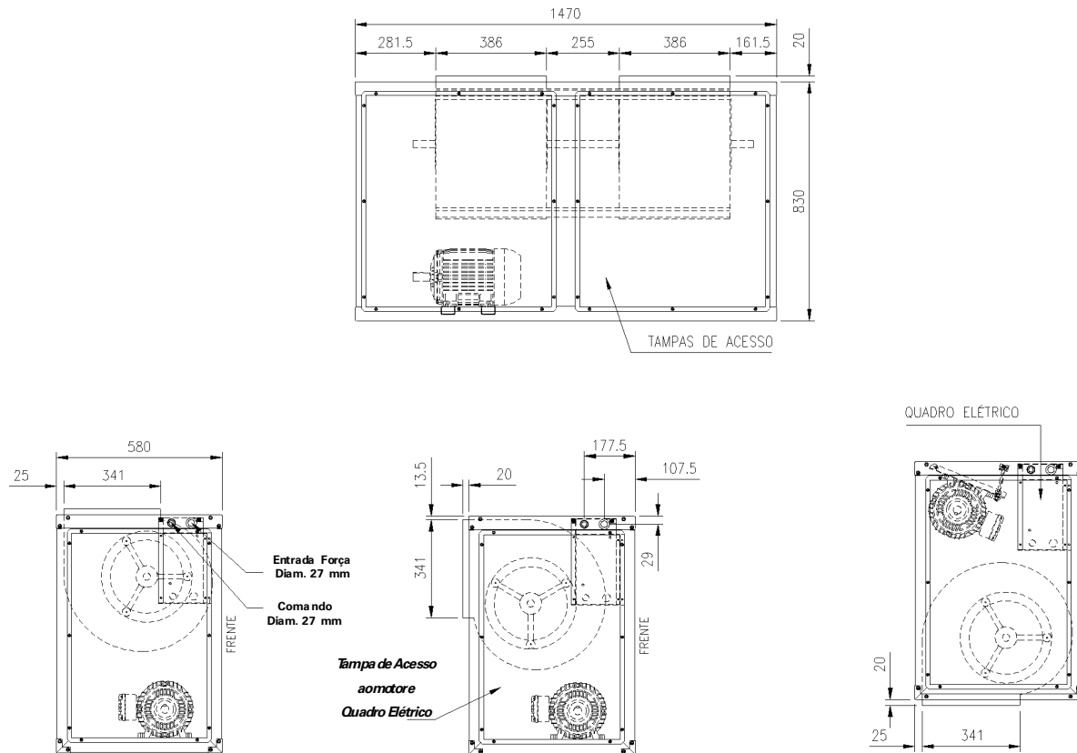
Fig. 13a - Descarga Vertical
