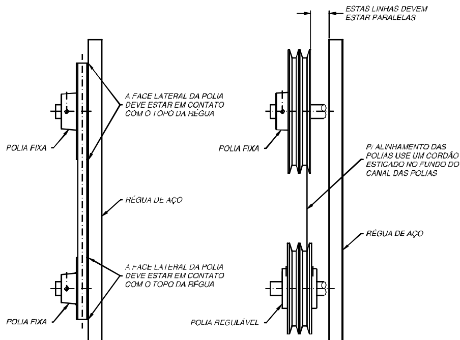
Fig. 04- Alinhamento das correias
