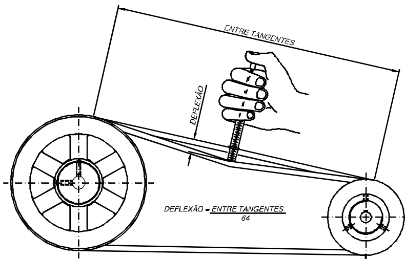
Fig. 06 - Ajuste da tensão da correia
